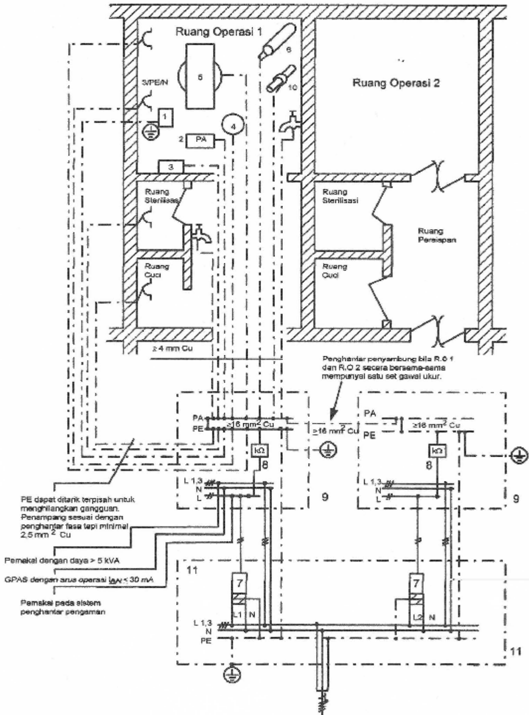
Gambar C.8.a.8) - 2 Contoh ekuiptensial di ruang operasi Catatan keterangan gambar C.8.a.8) - 2:
