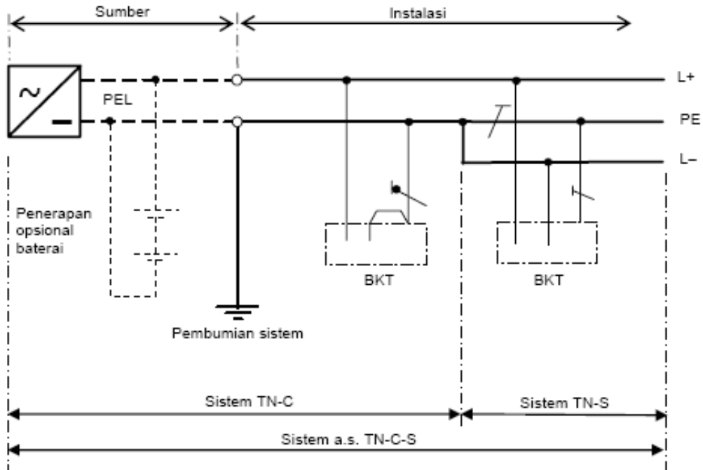
Gambar B.2.b.4).c) - A - Sistem a.s. TN-C-S
