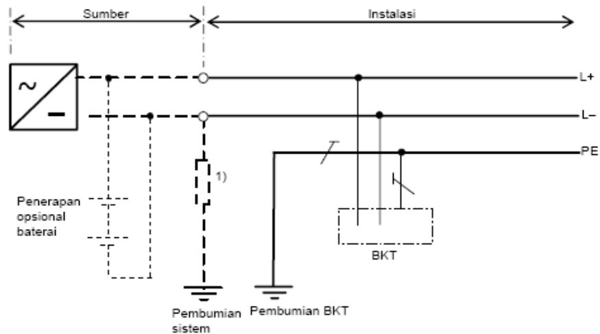
Gambar B.2.b.4).e) - A - Sistem a.s IT
