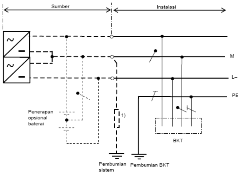
Gambar B.2.b.4).e) - B - Sistem a.s IT
