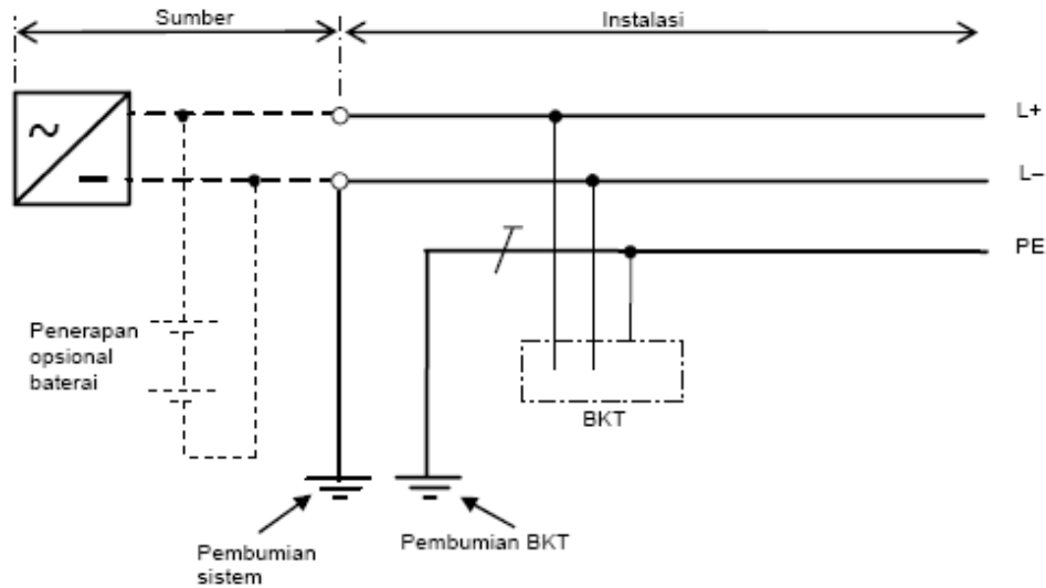
Gambar B.2.b.4).d) - A - Sistem a.s T.T
