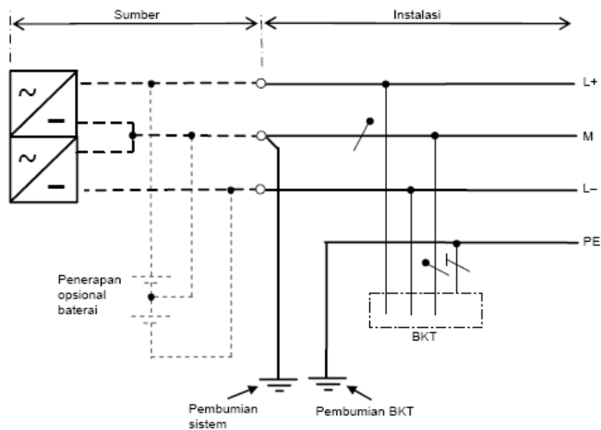
Gambar B.2.b.4).d) - B - Sistem a.s. TT
