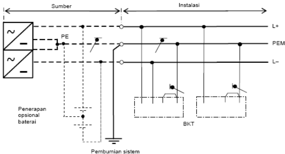
Gambar B.2.b.4).b) - B - Sistem a.s. TN-C
