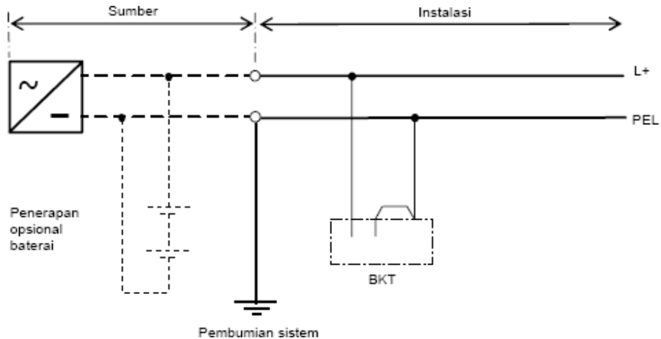
Gambar - B.2.b.4).b) - A
