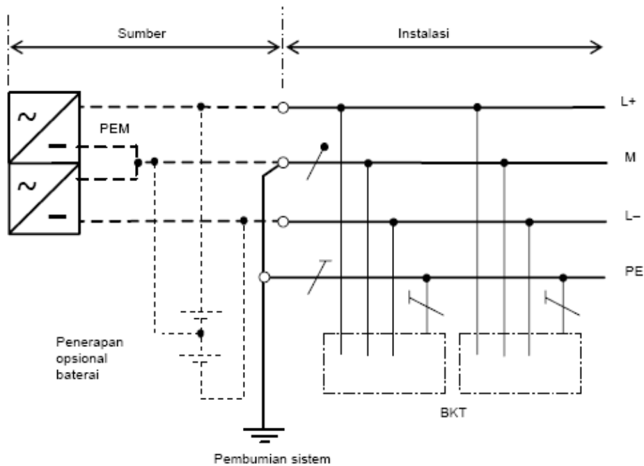
Gambar B.2.b.4).a) - B - Sistem a.s. TN-S
