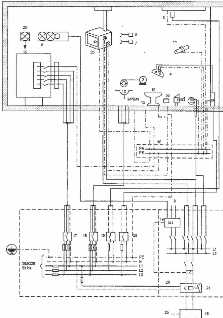
Gambar C.8.a.8) - 1 Contoh instalasi ruang operasi dengan equipotensial Catatan keterangan gambar C.8.a.8) - 1:
