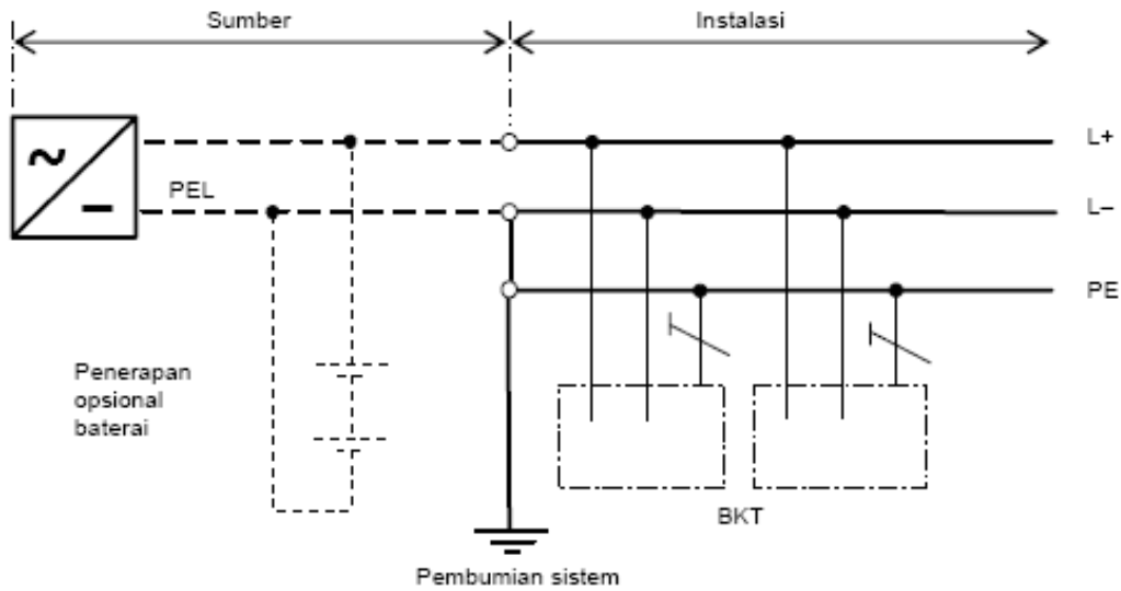
Gambar B.2.b.4).a) - A
