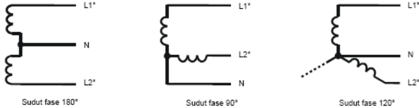
*Penomoran konduktor opsional Gambar B.2.a.1)-3 – Dwifase 3-kawat
