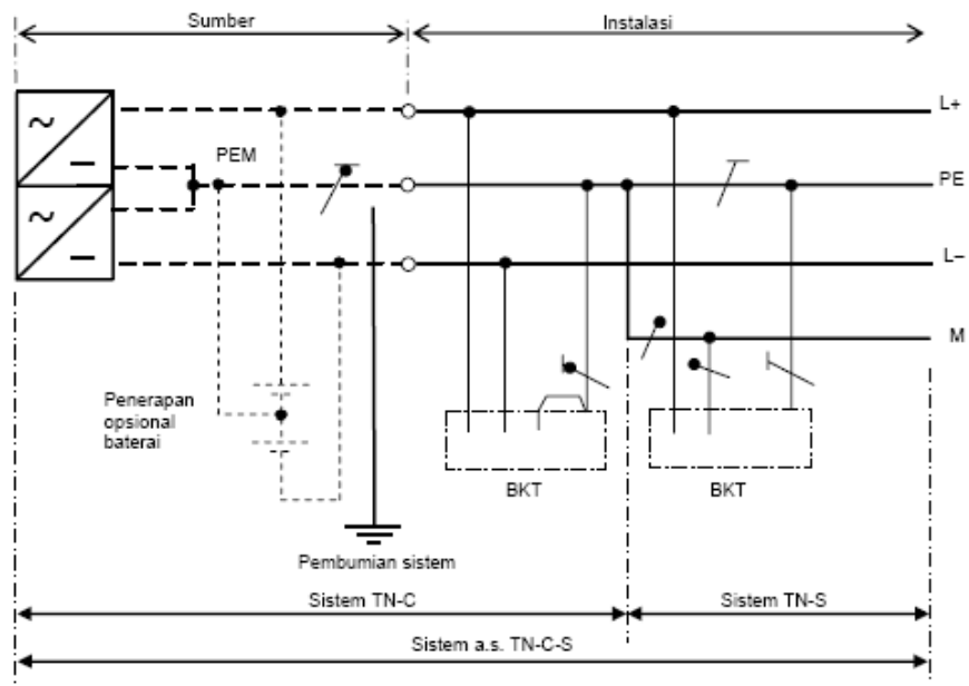
Gambar B.2.b.4).c) - B - Sistem a.s. TN-C-S
